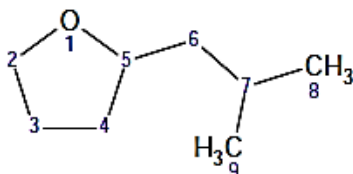
Рис.2. 2-Изобутитетрагидрофуран
